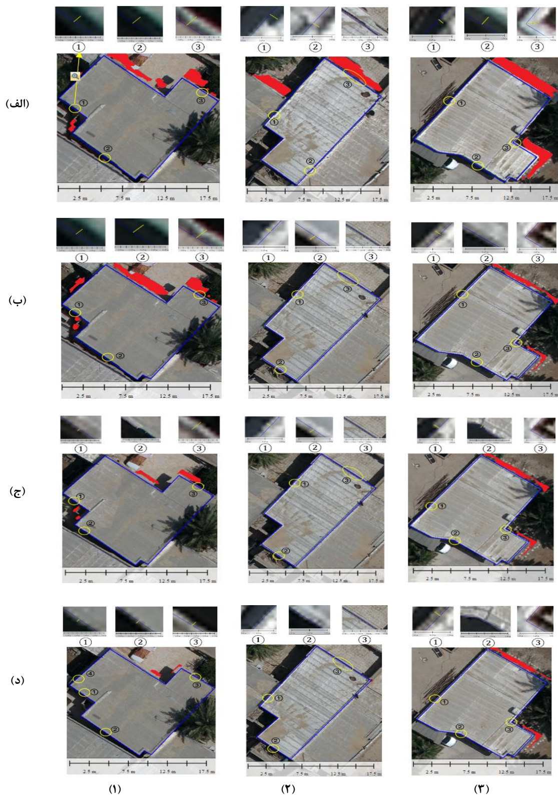
شکل ۱۰: ارزیابی دقت ارتوفتوموزاییک بدست آمده با استفاده از از چهار روش (الف) بر مبنای زاویه دید، (ب) بر مبنای فاصله از مرکز تصویربرداری، (ج) بر مبنای فاصله از نادیر و (د) روش پیشنهادی چندمعیاره مبنا در سه ناحیه (۱)، (۲) و (۳).
