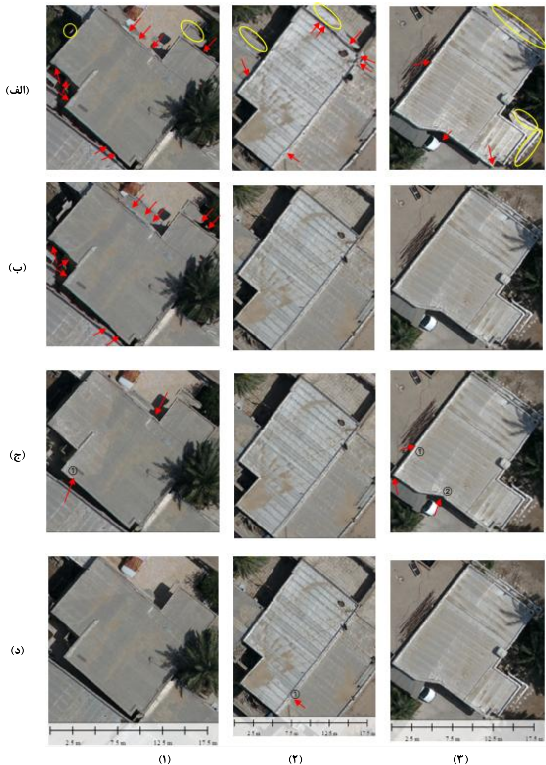
شکل ۸: ارتوفتوموزاییک‌های تولید شده در مجموعه داده اول در سه ناحیه (۱)، (۲) و (۳) با استفاده از چهار روش (الف) بر مبنای زاویه دید، (ب) بر مبنای فاصله از مرکز تصویربرداری، (ج) بر مبنای فاصله از ناوبر و (د) روش پیشنهادی چندمعیاره مبنای.
