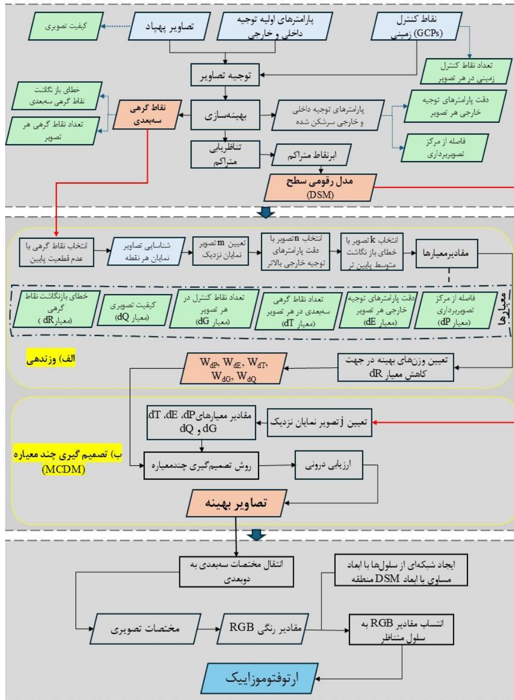
شکل ۴: روندنمای کلی روش پیشنهادی.
