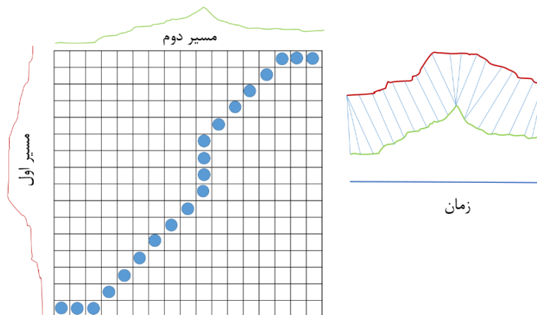
شکل ۱: سازوکار DTW [۱۸]
