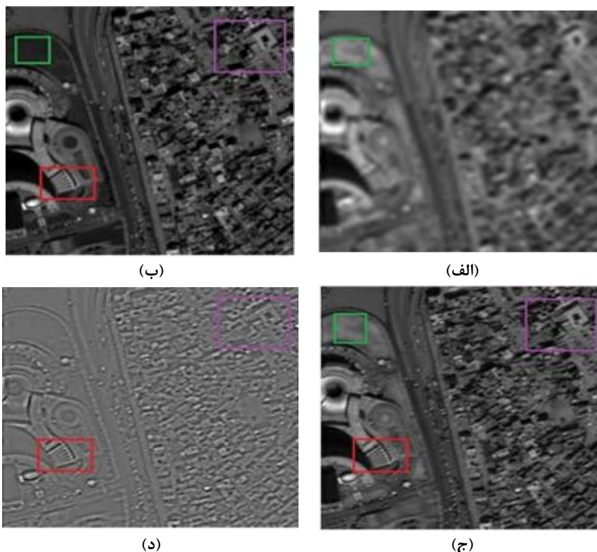
شکل ۴: عوارض بازسازی شده با استفاده از روش پیشنهادی، (الف): تصویر MS و هم اندازه با تصویر PAN، (ب): تصویر PAN، (ج): تصویر بازسازی شده MS، (د): عوارض ساختاری مستخرج (delta)
