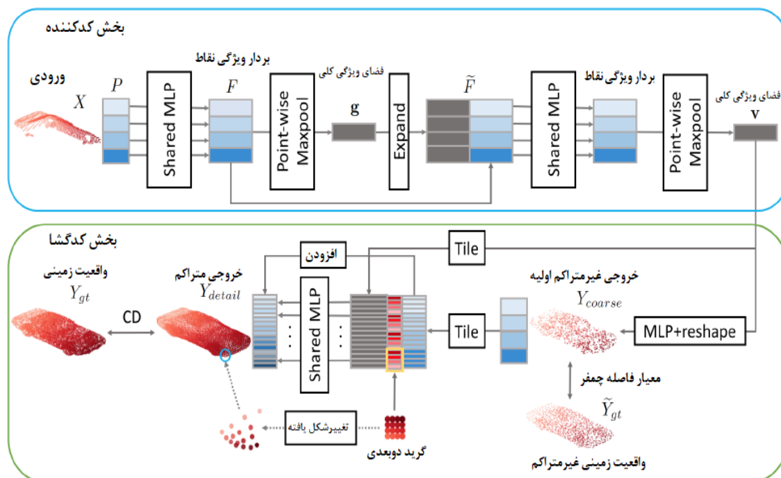
شکل ۵: شبکه یادگیری عمیق تکمیل‌کننده ابر نقاط سه‌بعدی [۲۲]
