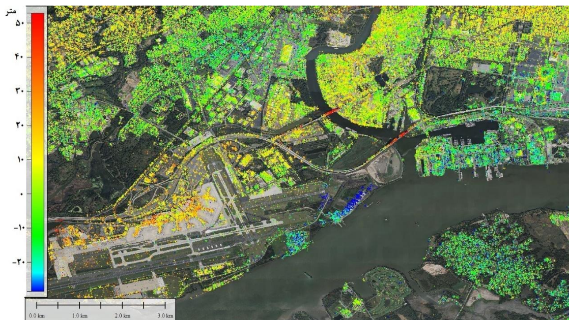
شکل ۶: ابر نقطه سه بعدی حاصل از پردازش تداخل سنجی راداری پراکنش گرهای دائمی تصاویر سنتینل-۱
