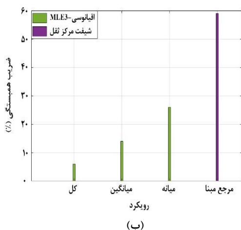
شکل ۵: پارامترهای آماری ارزیابی میان داده‌های حاصل از بازتعقیب‌گر بهینه و مشاهدات نوسان‌نگارمحل در گذر ۲۲۰ ماهواره جیسون-۳، (الف) RMSE ، (ب) ضریب همبستگی
