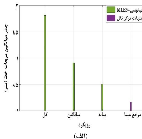
شکل ۵: پارامترهای آماری ارزیابی میان داده‌های حاصل از بازتعقیب‌گر بهینه و مشاهدات نوسان‌نگارمحل در گذر ۲۲۰ ماهواره جیسون-۳، (الف) RMSE ، (ب) ضریب همبستگی
