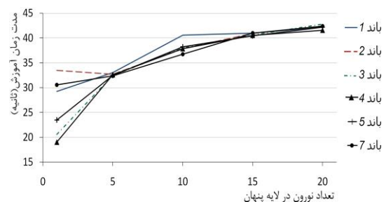
شکل ۱۱: روند تغییرات زمان یادگیری شبکه عصبی، به ازای افزایش تعداد نورون‌های لایه پنهان در باندهای ۷ و ۵ و ۴، ۳، ۲ و ۱ در جفت تصویر دوم.
