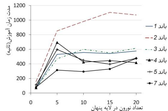
شکل ۱۰: روند تغییرات زمان یادگیری شبکه عصبی، به ازای افزایش تعداد نورون‌های لایه پنهان در باندهای ۷ و ۵ و ۴، ۳، ۲ و ۱ در جفت تصویر اول.
