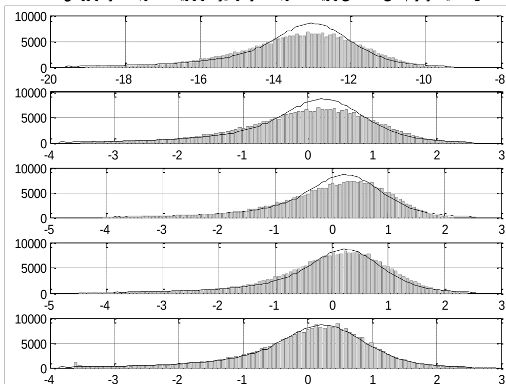
شکل ۹: هیستوگرام‌های داده‌های زاویه ۲۶ درجه (منحنی مشکی) و زاویه ۶۲ درجه (پلات خاکستری) پس از اعمال تصحیحات مرتبه ۱ و ۲ و ۳ و ۴
