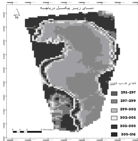
شکل (۶): دمای زیر پیکسل تصویر MODIS دریاچه ارومیه
