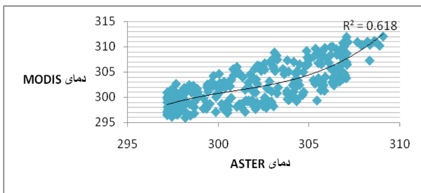
شکل (۸): نمودار ضریب تعیین بین دمای زیر پیکسل برحسب کلونین MODIS و ASTER
