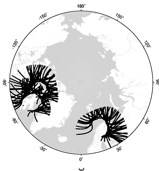
شکل ۲: موقعیت مکانی نقاط نفوذ یونسفری (الف: ایستگاه‌های کنترل و ب: ایستگاه‌های چک
