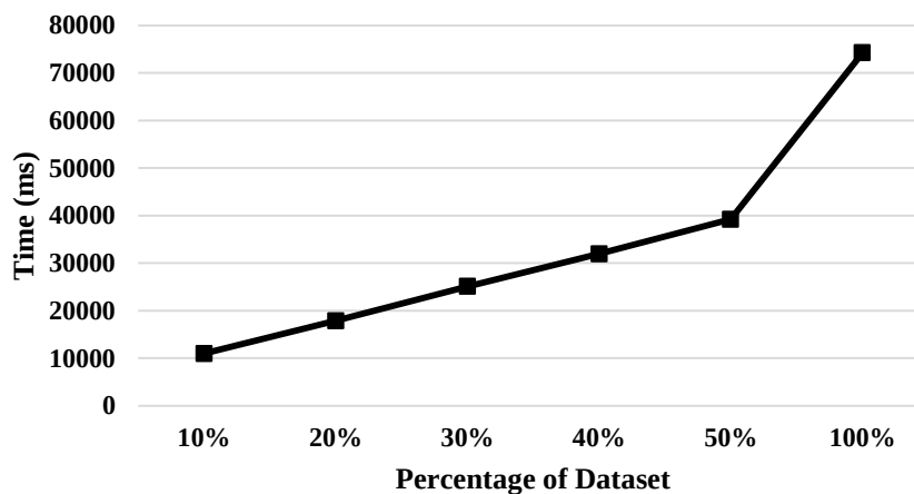
شکل ۷: زمان انجام پرس و جوی محدوده‌ای
