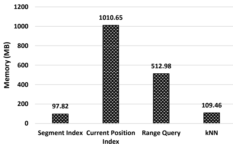
شکل ۸: میزان حافظه مصرفی در فرآیند شاخص‌گذاری و انجام پرس و جوها
