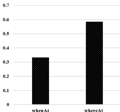
شکل ۳: الف. میانگین زمان لازم برای پرس‌وجو WhenAt و WhereAt ب. میانگین نسبت عملکرد پرس‌وجو
