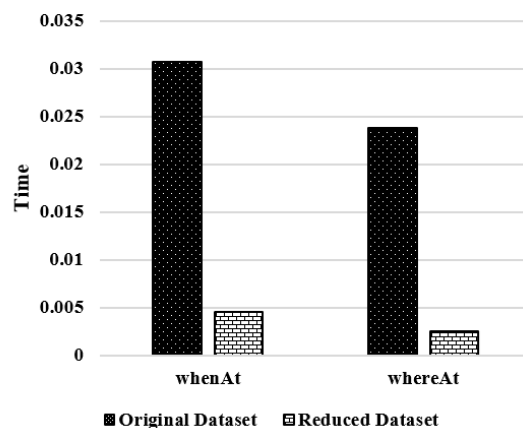
شکل ۳: الف. میانگین زمان لازم برای پرس‌وجو WhenAt و WhereAt ب. میانگین نسبت عملکرد پرس‌وجو
