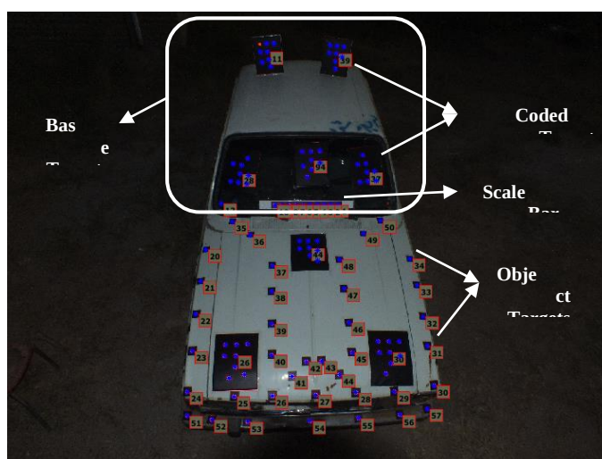
شکل ۳: تارگت‌های کد دار و تارگت‌های معمولی با پس زمینه قرمز، میله مقیاس مورد استفاده در پروژه.
