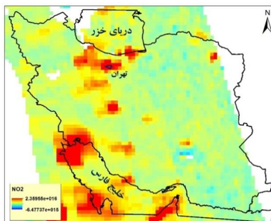
شکل ۳: نمونه‌ای از تصویر NO 2 سنجنده OMI
