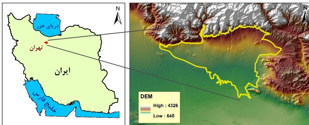
شکل ۱: موقعیت محدوده مطالعاتی (کلان شهر تهران)
