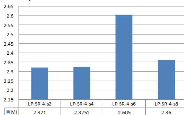
شکل ۱۰: ارزیابی تاثیر طول گام پنجره متحرک بر نتایج ادغام در روش LP-SR
