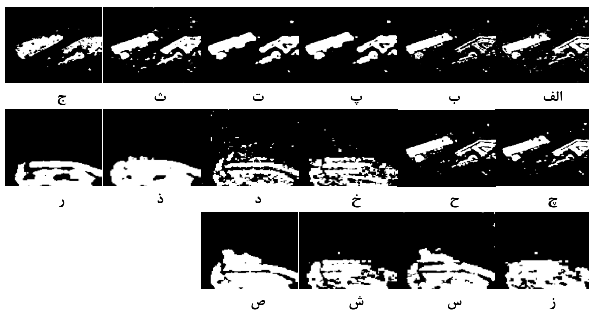
شکل ۱۳: خروجی الگوریتم جبری اختلاف تصاویر روی داده اول: الف) S1، ب) S2، پ) S3-1، ت) S4-1، ث) S3-2، ج) S4-2، د) S1، ذ) S3-1، ر) S4-1، ز) S3-2، س) S4-2، ش) S3-3، ص) S4-3
