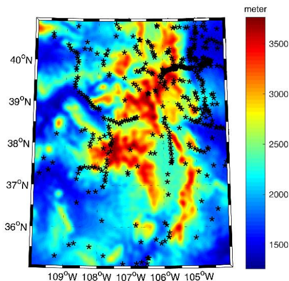
شکل ۱: توپوگرافی منطقه تست و نقاط ترازبایی با GPS موجود در آن منطقه
