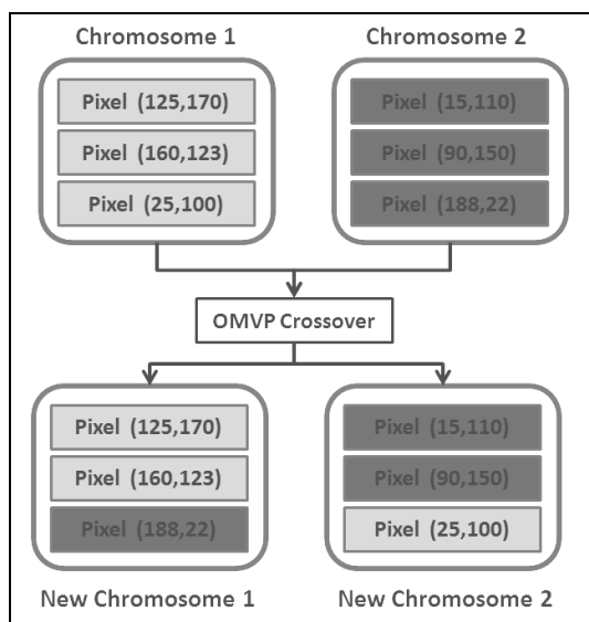
شکل ۴. فرایند تقاطع کروموزوم‌ها در مسئله OMVP
