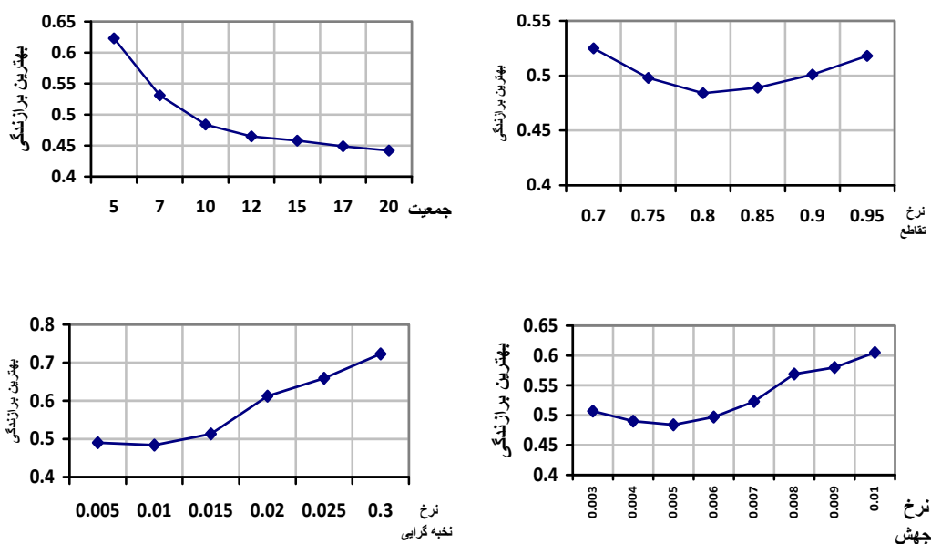
شکل ۹. ارزیابی نحوه تأثیر پارامترهای مختلف الگوریتم ژنتیک بر عدد برازندگی
