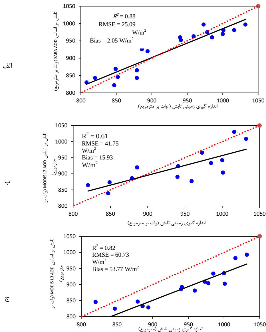
شکل ۵: اعتبارسنجی تابش های برآورد شده براساس داده های مختلف عمق اپتیکی هواویز (الف) SARA AOD (ب) MODIS L2 AOD (ج) MODIS L3 AOD در سایت چیتگر تهران سال ۲۰۱۳.
