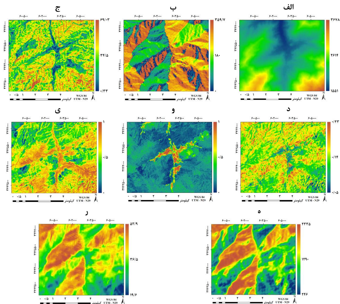
شکل ۱۱: نقشه پارامترهای محیطی برای روز ۲۴۸ سال ۱۴۰۱ الف) ارتفاع (متر)، ب) جهت شیب (درجه)، ج) شیب (درجه)، د) آلودگی، و) سبزی، ی) رطوبت سطح، ه) تابش تجمعی موثر رسیده به سطح و ر) دمای سطح بدست آمده از لندست
