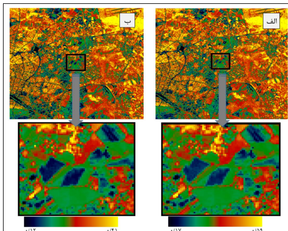
شکل ۵: میزان آلودگی محاسباتی با استفاده از سنجنده OLI و روش‌های ساده فاقد تصحیح جوی (الف) و تصحیح شده به روش تاسومی (ب) می‌باشند
