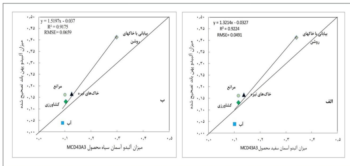
شکل ۶: میزان همبستگی و خطای حاصل از آلبیدو تصحیح شده و محصول MCD43A3 در شرایط مفروض الف) آسمان سفید و ب) آسمان سیاه مربوط به میانگین ۲۵۰ نقطه مشاهداتی در کاربری‌های مختلف
