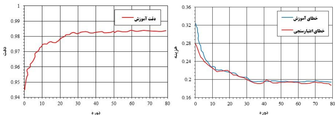
شکل ۶: منحنی تکرار بر روی مجموعه داده تحقیق با استفاده از روش پیشنهادی، محور افقی: تعداد تکرار، محور عمودی: اختلاف اندازه‌گیری‌ها. شکل راست: خطای آموزش و خطای اعتبارسنجی در ۷۹ تکرار (بهترین مدل برای مجموعه داده تحقیق)، شکل چپ: منحنی دقت آموزش مدل
