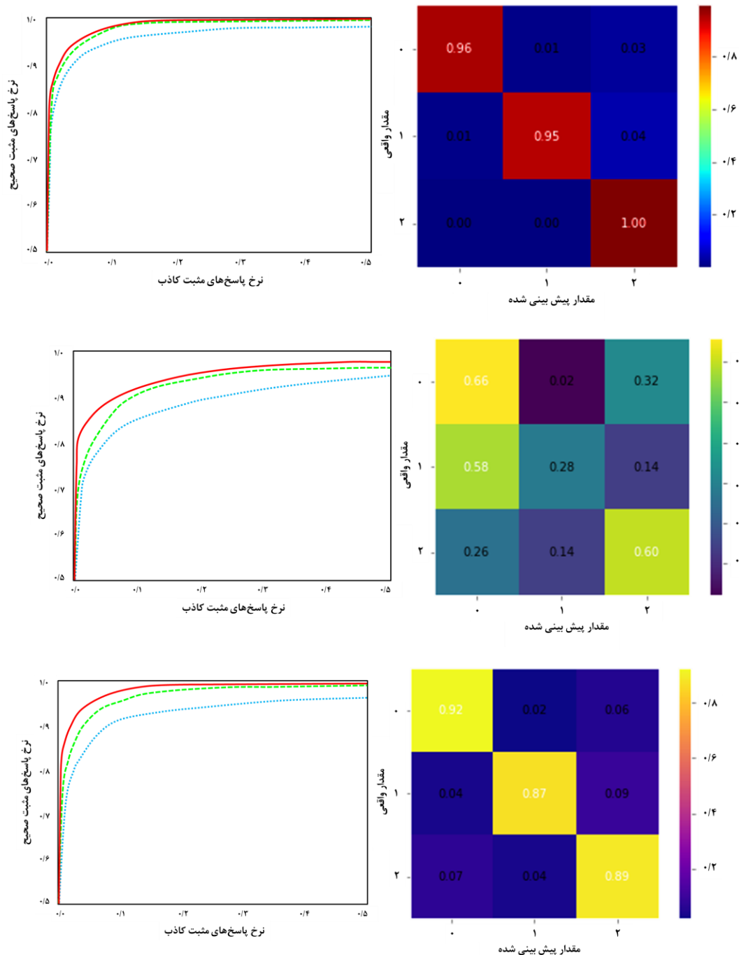
شکل ۶: ماتریس ابهام و منحنی مشخصه عملکرد سیستم مربوط به تمام نمونه‌های آزمایشی به تفکیک روش‌های مورد استفاده. سطر اول تا سوم به ترتیب معرف روش MultiCloud-Net ترکیب ویژگی‌ها و تلفیق ویژگی‌های کانوولوشنی چندمقیاسه می‌باشد. کلاس صفر، یک و دو به ترتیب معرف کلاس ابر، سایه ابر و پس‌زمینه می‌باشند. در منحنی‌های مشخصه عملکرد سیستم، رنگ قرمز، سبز و آبی به ترتیب مربوط به کلاس پس‌زمینه، ابر و سایه ابر می‌باشند.
