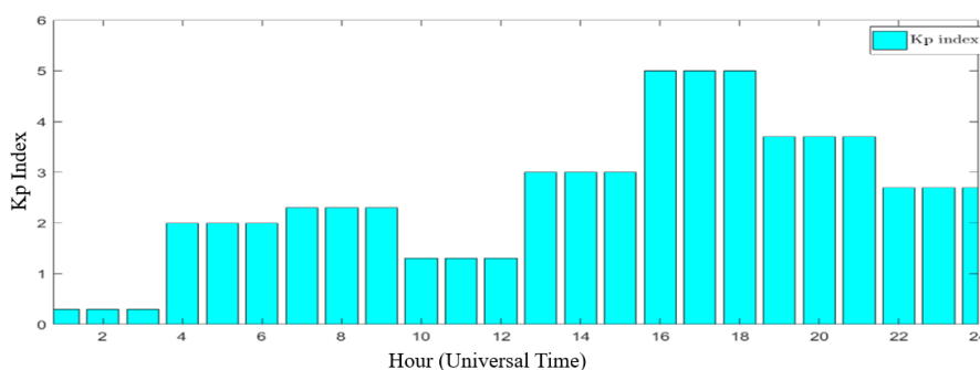
شکل ۵: شاخص ژئومغناطیسی بین‌المللی Kp index سه ساعته برای دهم ماه ژوئن سال ۲۰۱۷
