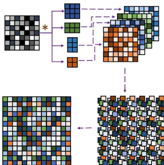
شکل ۵: نحوه دو برابر کردن ابعاد نقشه‌های ویژگی در طی مرحله کدگذاری
