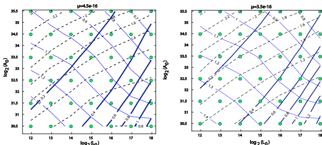
شکل ۵: مقدار \mu, \mu^* (تصویر بالا (۵-الف)) و دو معیار خطای N_2^{stres}, N_2^{geodic} به صورت تابعی از \mu با در نظر گرفتن
