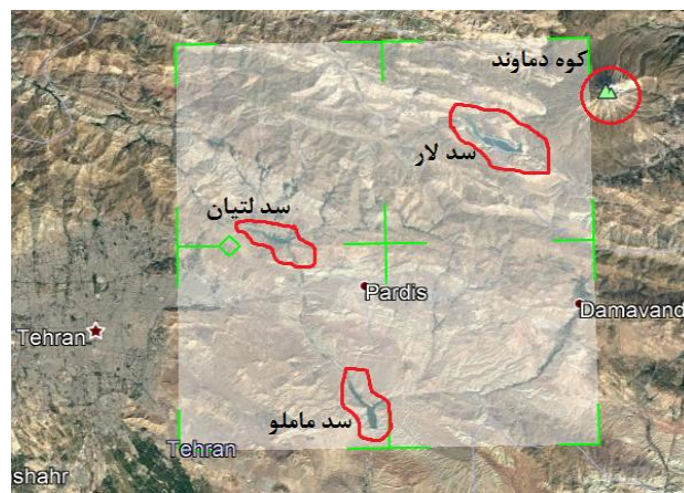
شکل ۵: موقعیت کوه دماوند و سدهای موجود در منطقه در تصویر سنجنده SLSTR ماهواره سنتینل-۳A
