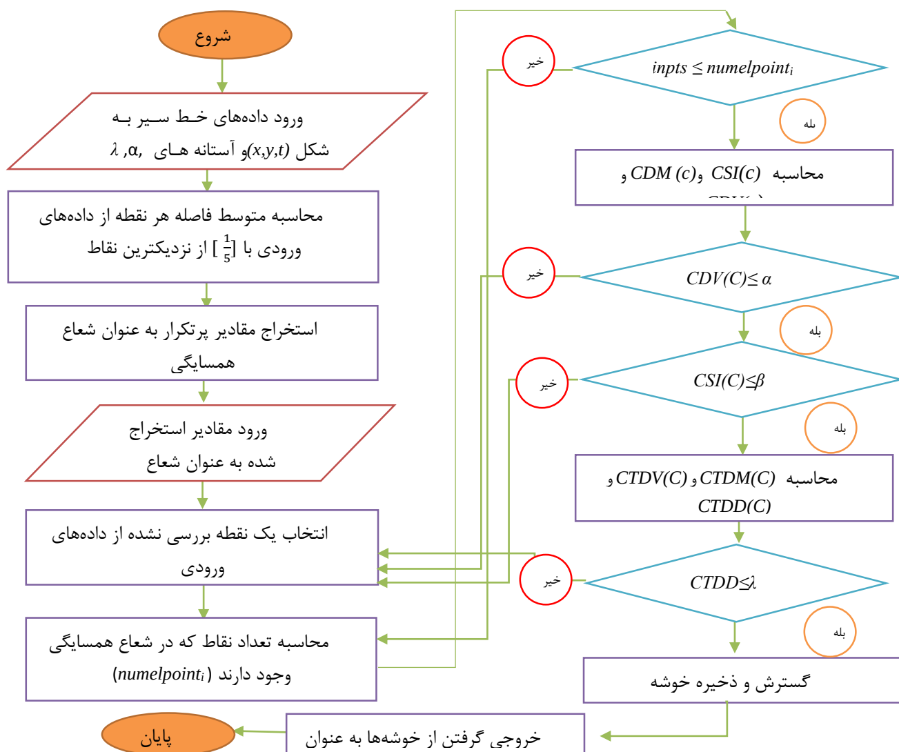
شکل ۲: روندنمای روش پیشنهادی (VDBSTCAN)
