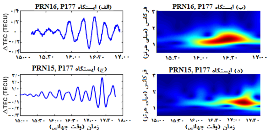
شکل ۱۰: سری زمانی \Delta TEC و آنالیز فرکانسی PRN15 و PRN16 مشاهده شده در ایستگاه P177 بین بازه زمانی ۱۵:۰۰ الی ۱۸:۰۰ به وقت جهانی
