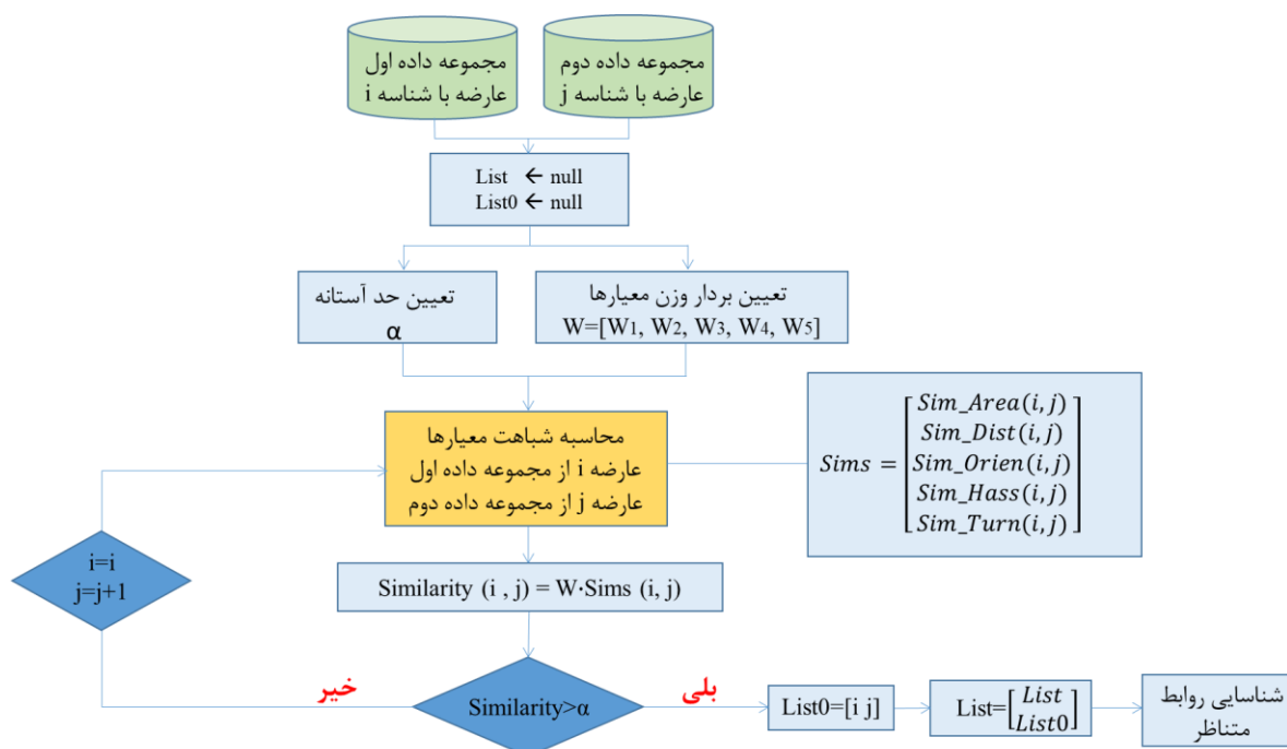
شکل ۲: فلوچارت الگوریتم تناظریابی مورد استفاده
