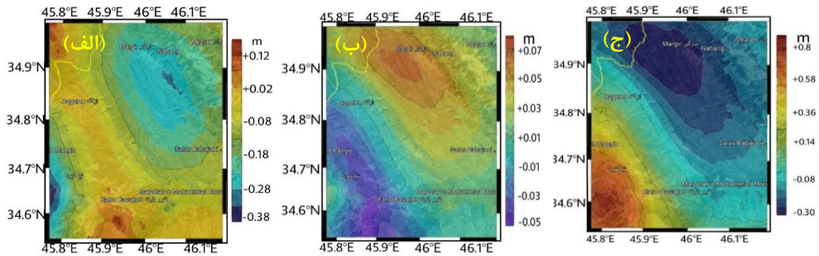
شکل ۵- (الف) مؤلفه میدان جابجایی در راستای شمالی-جنوبی و (ج) مؤلفه میدان جابجایی در راستای شرقی-غربی، (ب) مؤلفه میدان جابجایی در راستای شمالی-جنوبی و (ج) مؤلفه میدان جابجایی در راستای شرقی-غربی
