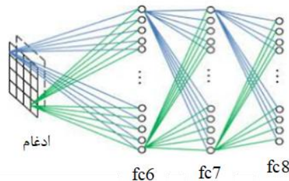
شکل ۲: عملیات لایه ادغام [۲۰]
