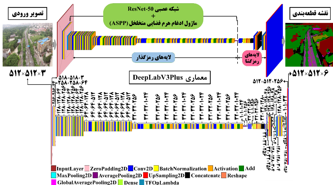
شکل ۳: معماری DeepLabV3Plus طراحی شده (ابعاد تصاویر ورودی 512 \times 512 \times 3 و ابعاد نقشه قطعه بندی خروجی 512 \times 512 \times 7 ).
