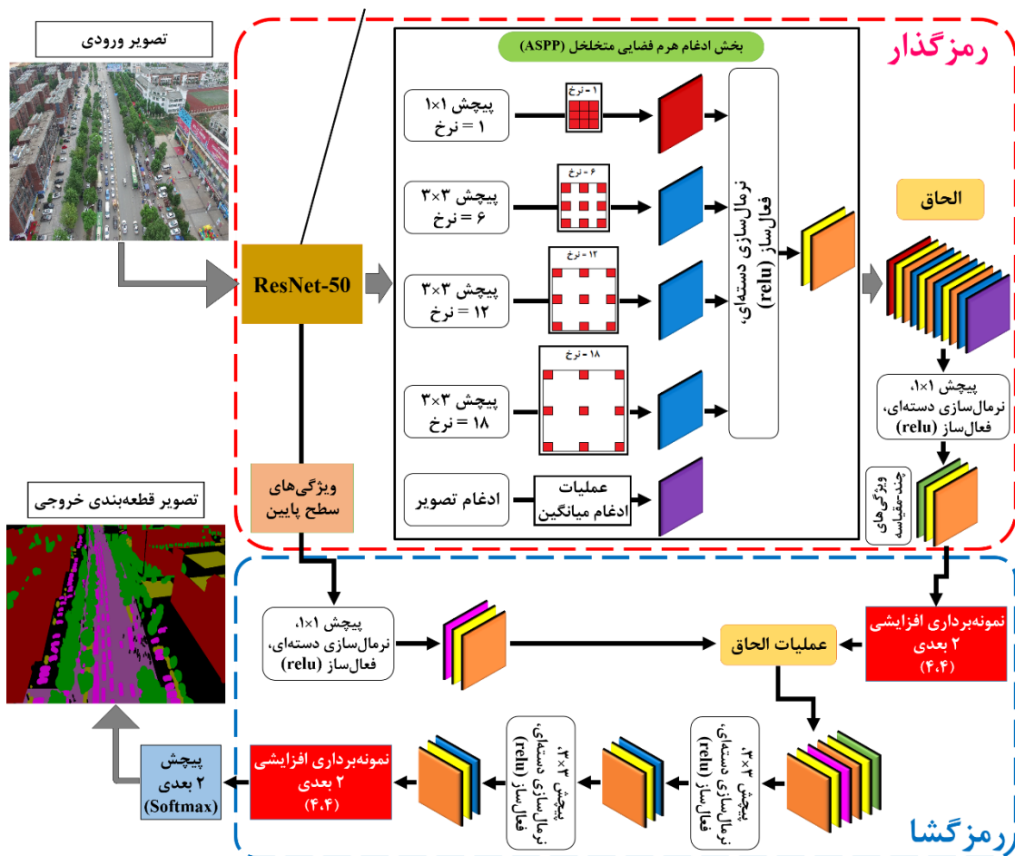
شکل ۲: معماری DeepLabV3+ با شبکه از قبل آموزش دیده ResNet-50
