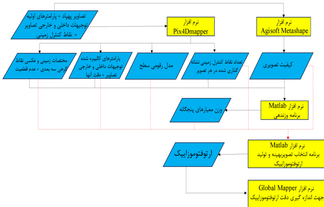
شکل ۷: روندنمای اجرایی روش پیشنهادی در تولید ارتوفتوموزائیک.
