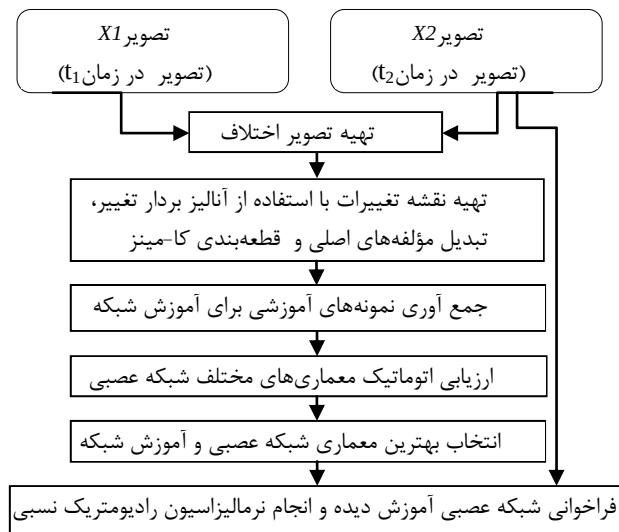
شکل ۲: فلوچارت روش پیشنهادی در تحقیق حاضر.
