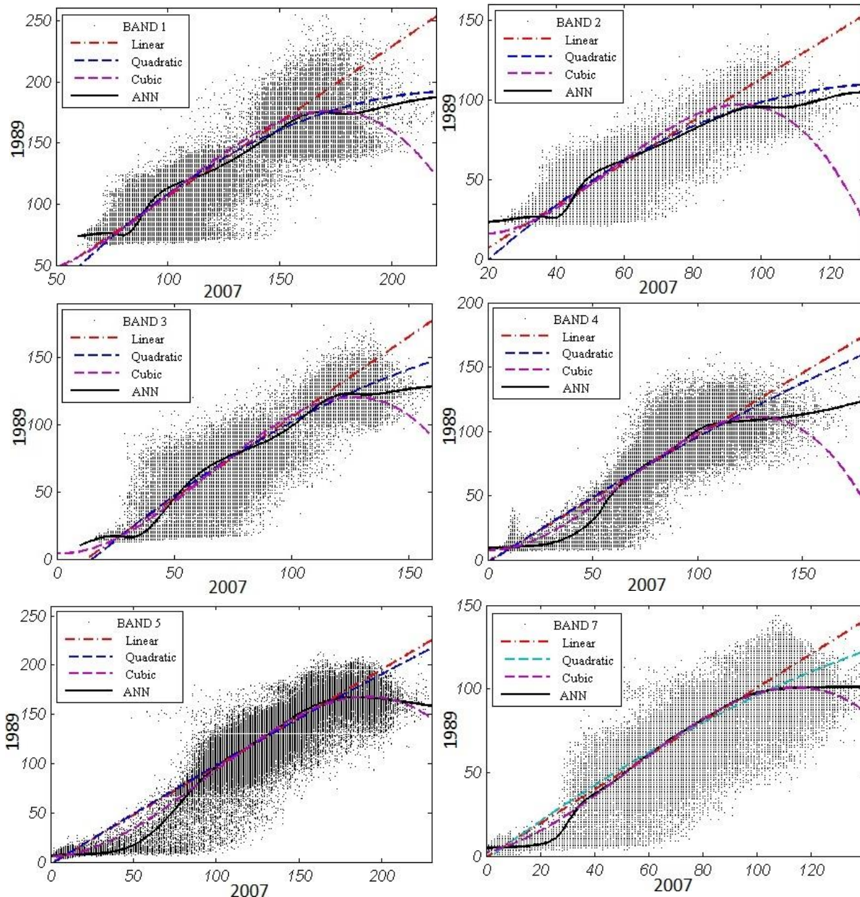
شکل ۳: توزیع درجات خاکستری پیکسل‌های تغییر نیافته در دو تصویر هدف و مرجع، در باندهای ۱، ۲، ۳، ۴، ۵ و ۷ به همراه مدل‌های خطی درجات اول، دوم و سوم و همچنین مدل غیر خطی حاصل از شبکه عصبی برازش داده شده.
