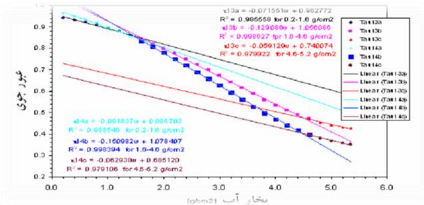
شکل ۱: نمودار میزان قابلیت عبور جو برای مقادیر مختلف بخار آب جو
