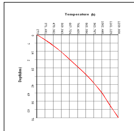
شکل ۶. ژئوترم محاسبه شده برای رئولوژی سرد که در مدل خزشی استفاده می‌شود. محور افقی درجه حرارت برحسب کلون را نشان می‌دهد و محور قائم عمق برحسب کیلومتر است.
