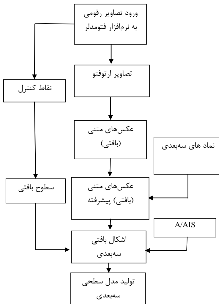
شکل ۴: الگوریتم توسعه (A / AIS) برای تولید مدل سطحی سه بعدی به کمک نرم افزارهای اتوکلد و فتومدلر را نشان می دهد
