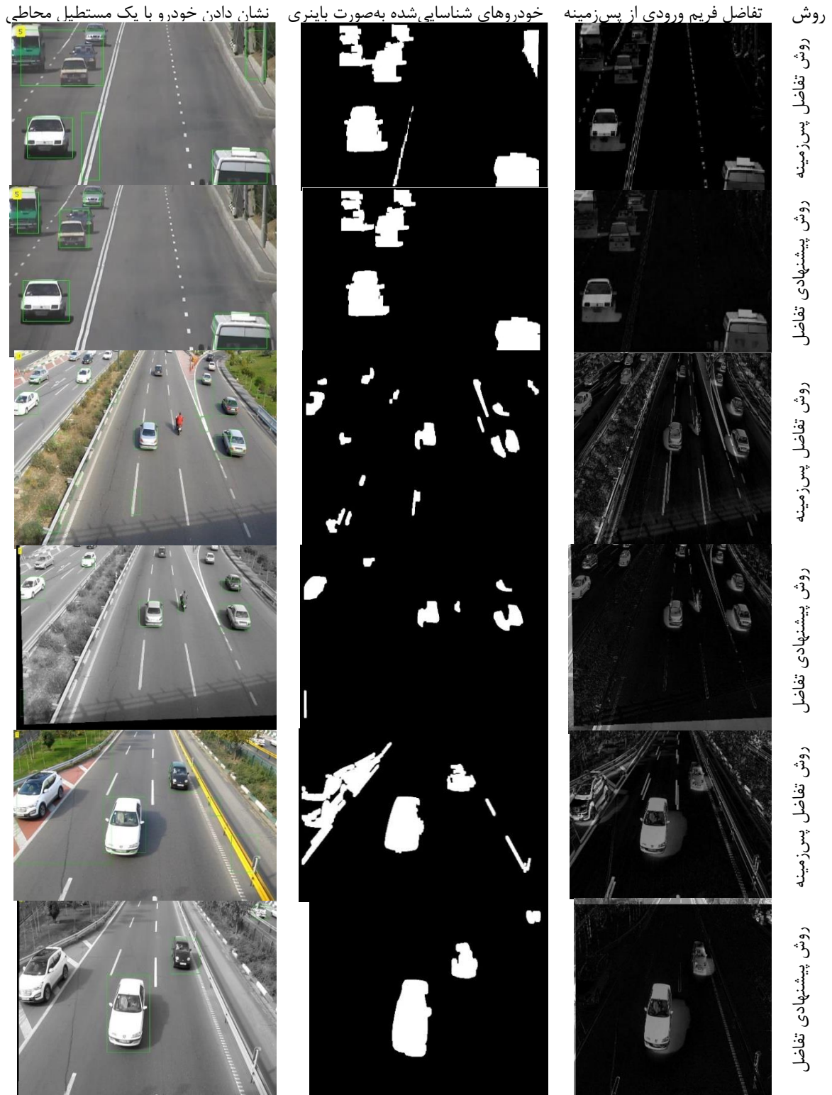
شکل ۶: ستون اول) تفاضل فریم‌های متوالی از تصویر پس زمینه در هر دو حالت با ثابت و بدون ثابت. ستون دوم) خودروهای شناسایی شده به صورت باینری در هر دو حالت با ثابت و بدون ثابت. ستون سوم) نشان دادن خودرو با یک مستطیل محاطی در هر دو حالت با ثابت و بدون ثابت
