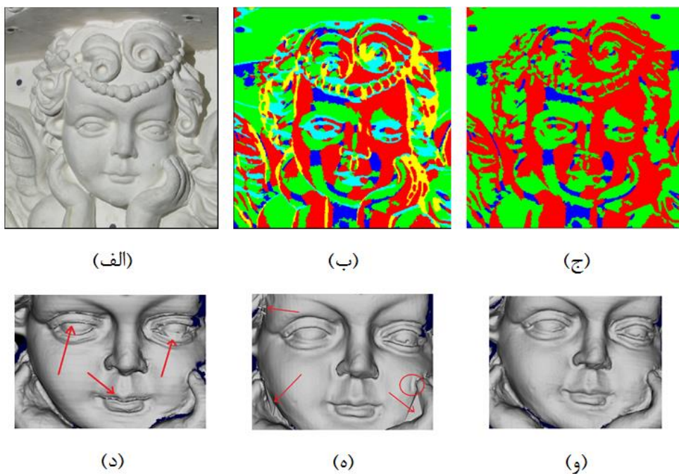
شکل ۷: ارزیابی کیفیت. (الف) تصویری از مجسمه. (ب) طبقه بندی سطوح و لبه ها. (ج) ادغام سطوح و لبه ها با جهت الگوی مشابه. (د) مدل سه بعدی به دست آمده با الگوی فرینج افقی. (ه) مدل سه بعدی بدست آمده با الگوی فرینج عمودی. (و) مدل سه بعدی به دست آمده با روش سه بعدی. جهت فلشها در (د) و (ه) نشان دهنده مشکلات بازسازی سه بعدی به علت جهت نامناسب الگوی نگاشت یافته می باشد.
