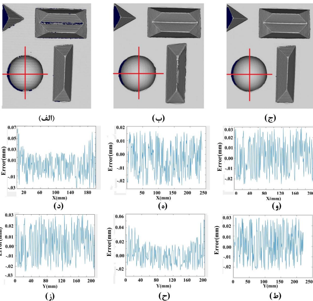
شکل ۶: نتایج آزمون و بررسی. (الف) مدل سه بعدی با استفاده از الگوی فرینج عمودی. (ب) مدل سه بعدی با استفاده از الگوی فرینج افقی. (ج) مدل سه بعدی با استفاده از روش پیشنهادی. (د-ط) خطای حاصل از مقایسه داده اندازه‌گیری در راستای مقاطع عرضی مشخص شده با دایره ایده آل.
