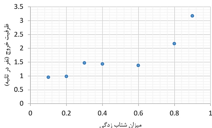
شکل ۱۴: تغییرات میزان ظرفیت خروج با تغییرات شتاب‌زدگی.
