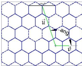
شکل ۷: پارامتر زاویه حرکت نسبت به خروجی
