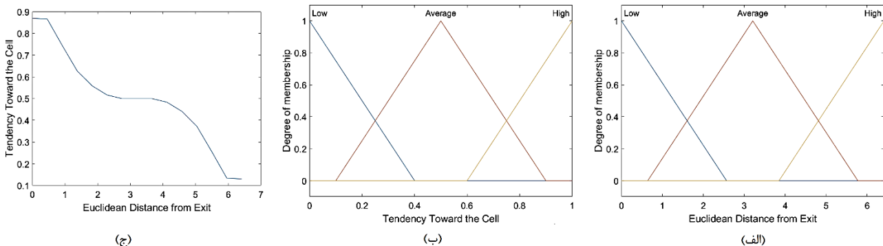
شکل ۴: نمایش سیستم فازی برای فاصله از خروجی. (الف) تابع عضویت برای فاصله از خروجی، (ب) تابع عضویت فازی برای میزان تمایل به رفتن به سلول، (ج) نتیجه‌ی سیستم فازی بر اساس قوانین ذکر شده
