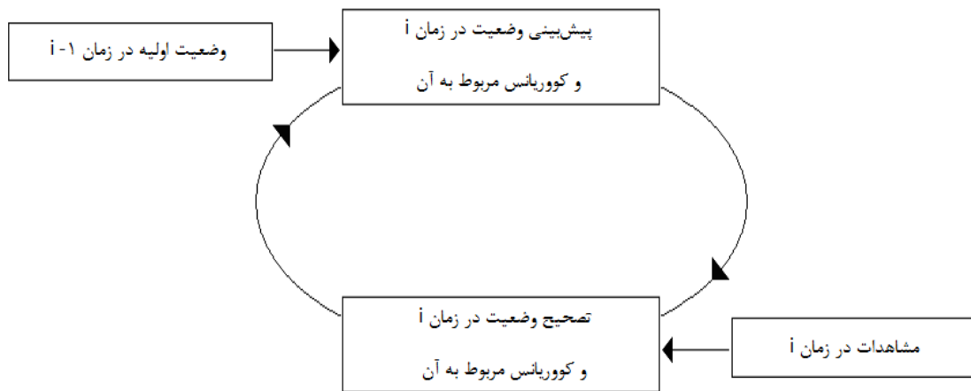
شکل ۸: مراحل فیلتر کالمن
