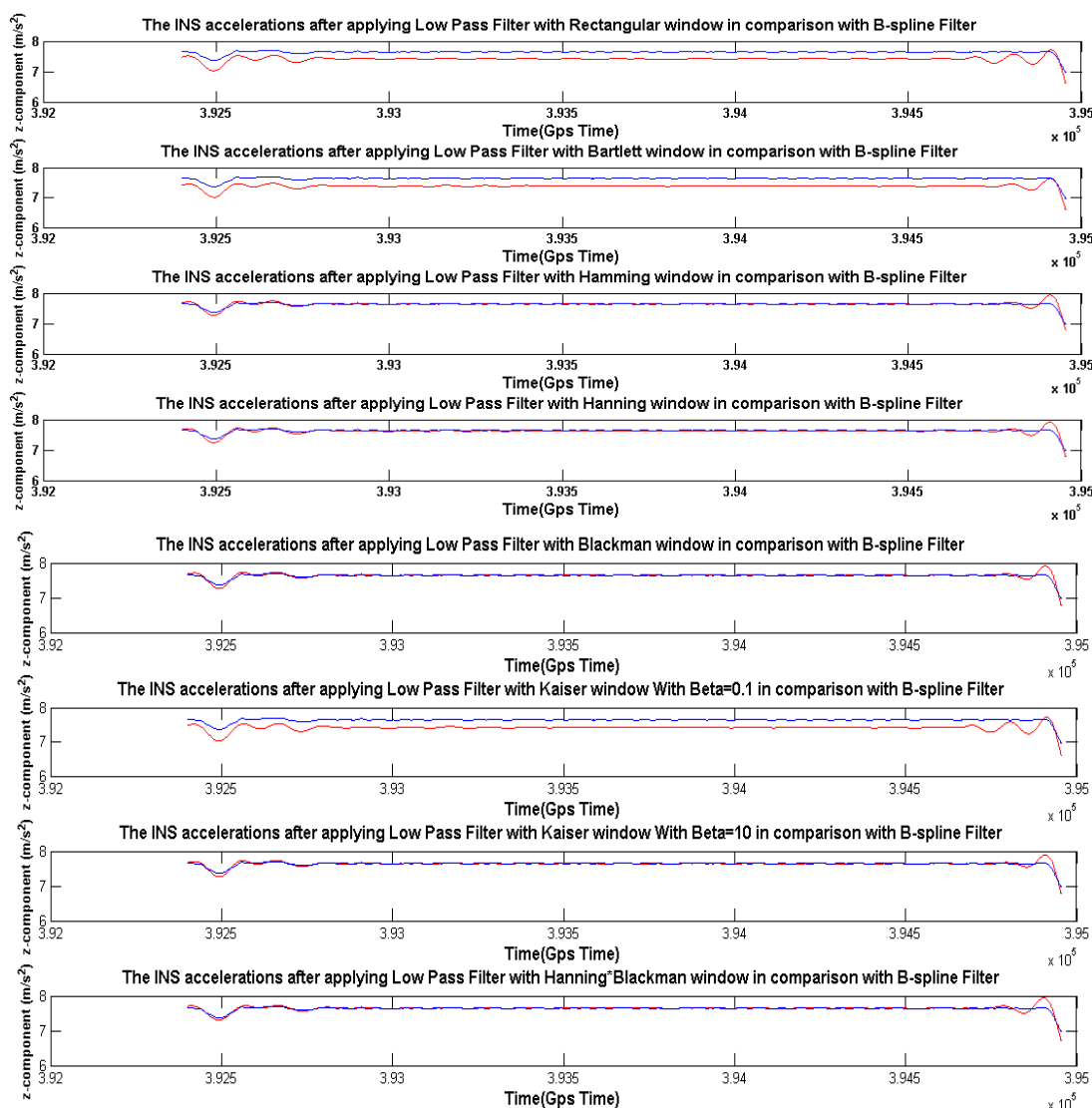
شکل ۱۳: شتاب INS بعد از اعمال فیلتر پایین‌گذر با پنجره‌های مختلف (رنگ قرمز) و فیلتر B-spline (رنگ آبی)
