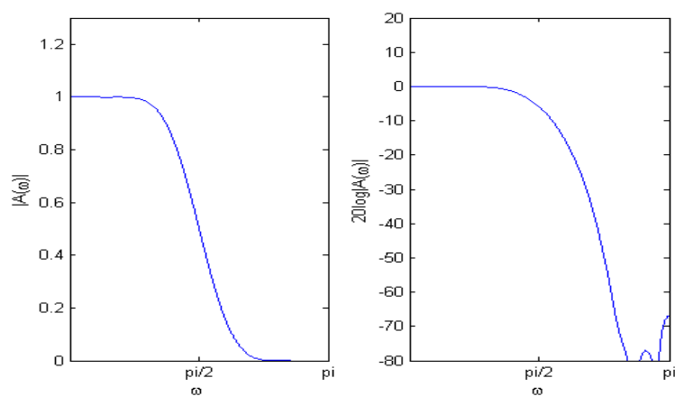
پنجره حاصلضرب پنجره‌های هنینگ و بلکمن
