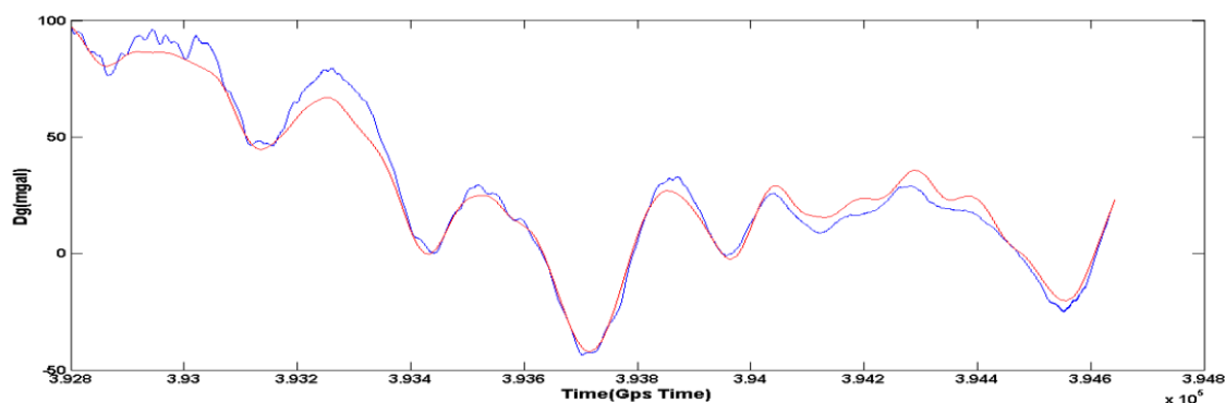
شکل ۲۲: نوسان شتاب ثقل اسکالر محاسبه شده با استفاده از فیلتر پایین‌گذر با پنجره حاصلضرب پنجره‌های هنینگ و بلکمن
