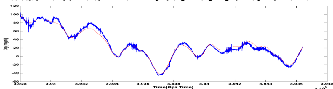
شکل ۲۳: نوسان شتاب ثقل اسکالر محاسبه شده با استفاده از فیلتر پایین‌گذر با پنجره کایزر با پارامتر \beta = 0.1 بعد از اعمال
