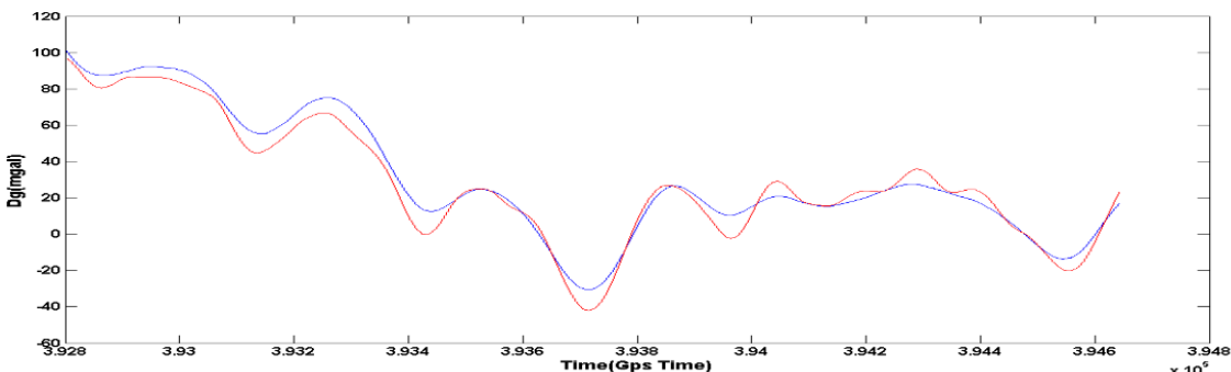
شکل ۲۵: نوسان شتاب ثقل اسکالر محاسبه شده با استفاده از فیلتر B-spline بعد از اعمال فیلتر کالمن
