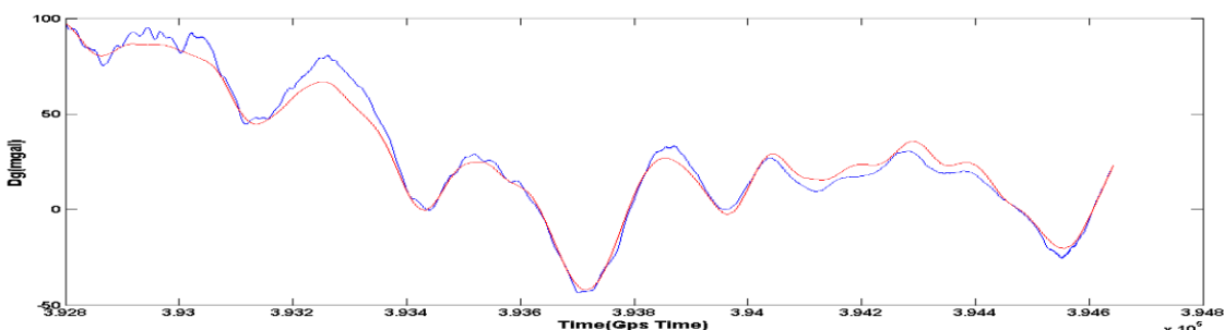
شکل ۲۴: نوسان شتاب ثقل اسکالر محاسبه شده با استفاده از فیلتر پایین‌گذر با پنجره کایزر با پارامتر \beta = 10 بعد از اعمال
