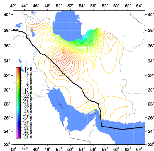
شکل ۷. الگوی تغییر شکل ارتفاعی در کشور حاصل از مشاهدات GPS شبکه موردی مرسوم به ایران سراسری. نتایج نمایش داده شده در ۱۰ ۷ ضرب شده است. امتداد مرز صفحات تکتونیکی عربی و اوراسیا با خط مشکی‌رنگ توپر نمایش داده شده است.
