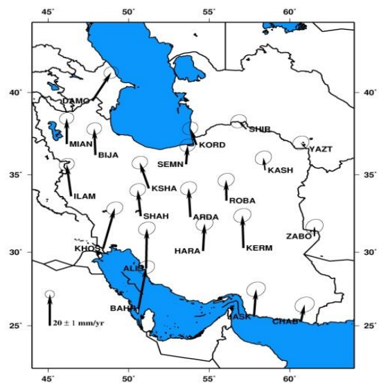
شکل ۵. میدان سرعت شبکه ایران بین سال‌های ۲۰۰۵-۲۰۰۱ در فریم اوراسیا. بیضی‌های خطای موقعیت نقاط در سطح اطمینان ۹۵ درصد ترسیم شده‌اند.
