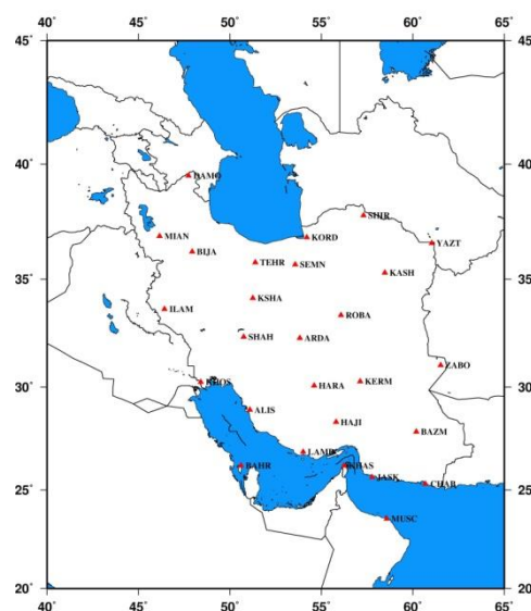
شکل ۱. ایستگاه‌های GPS موردی شبکه موسوم به ایران سراسری. نام اختصاری هر ایستگاه در کنار محل ایستگاه نمایش داده شده است.
