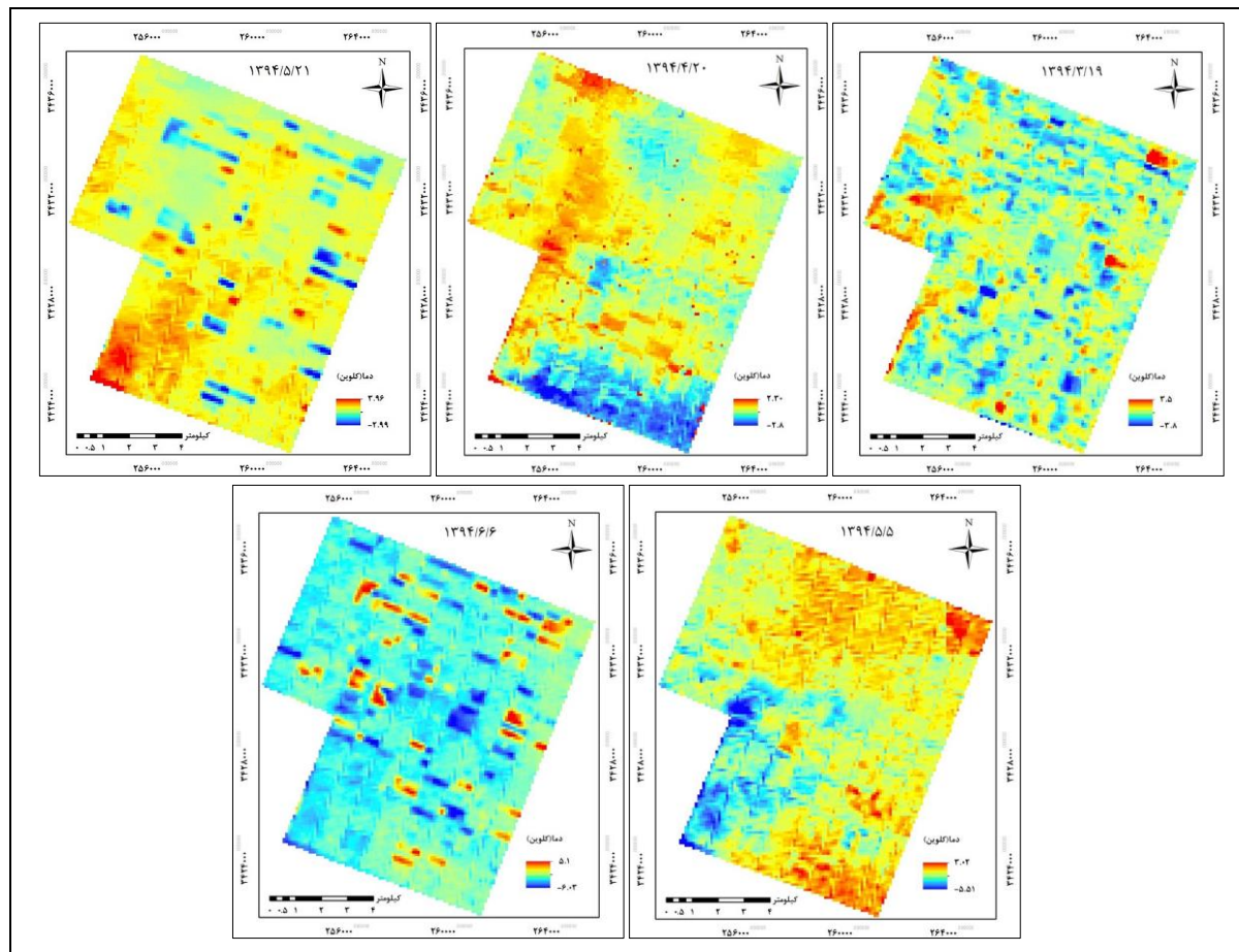
شکل ۷: اختلاف دمای سطح پیش‌بینی شده و دمای سطح مشاهده شده برای تاریخ‌های مختلف (کلوین)
