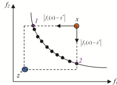
شکل ۲: تعبیر مفهوم وزن در الگوریتم MOEA/D، x
