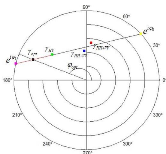
شکل ۳: نمایش موقعیت همدوسی حجمی بهینه بر روی خط همدوسی در مقایسه با همدوسی مورد استفاده در روش مرسوم سه مرحله‌ای در داده QP . مقادیر همدوسی در پایه‌های پائولی به ترتیب با رنگ‌های آبی، قرمز و سبز نشان داده شده است. همدوسی زمینی با نام e^{i\phi_0} و با رنگ زرد نمایش داده شده است. همدوسی حجمی بهینه حاصل از روش ESPO با رنگ مشکی و با عنوان \gamma_{opt} دیده می‌شود [۱۲].
