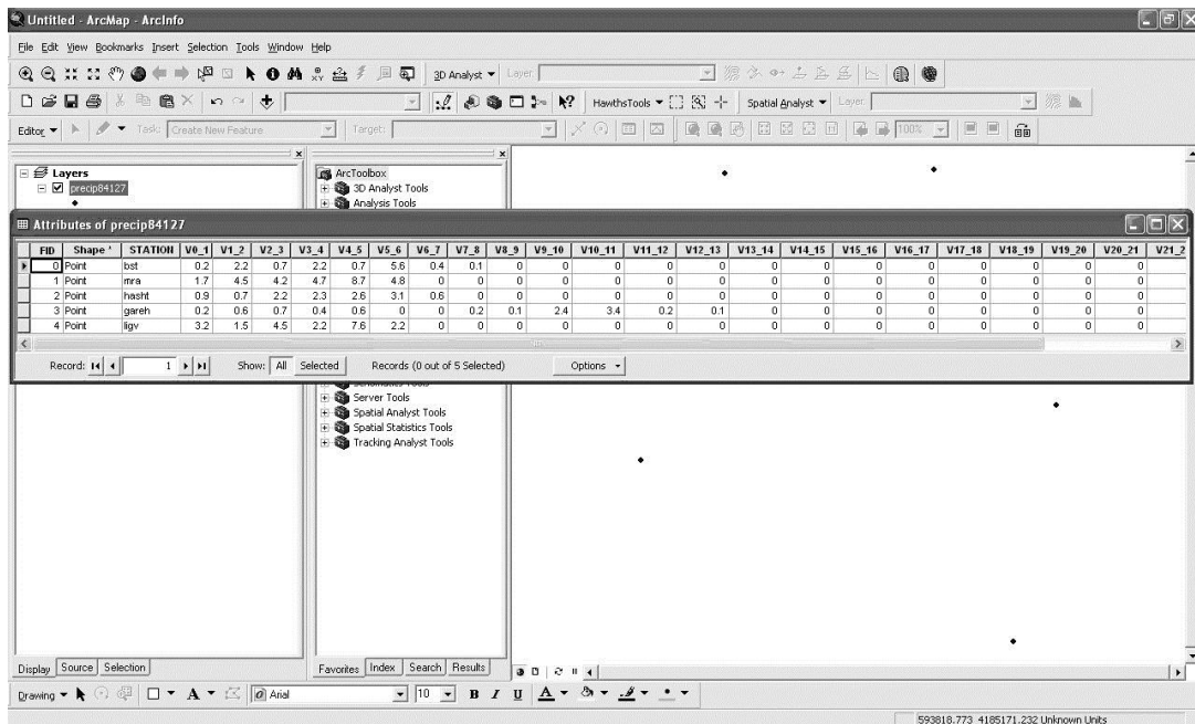
شکل ۲. شدت‌های یک‌ساعته ایستگاه‌ها در محیط GIS
