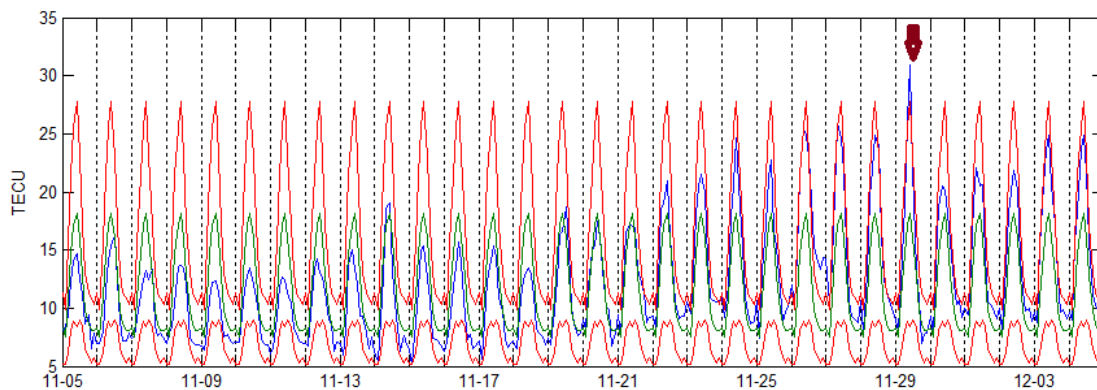
شکل ۱۳: نتایج بررسی تغییرات TEC نقطه‌ای از شبکه با مختصات ۳۲/۵ درجه شمالی و ۵۰ درجه شرقی، محور افقی نشان دهنده تاریخ و محور عمودی مقادیر TEC برحسب TECU است.
