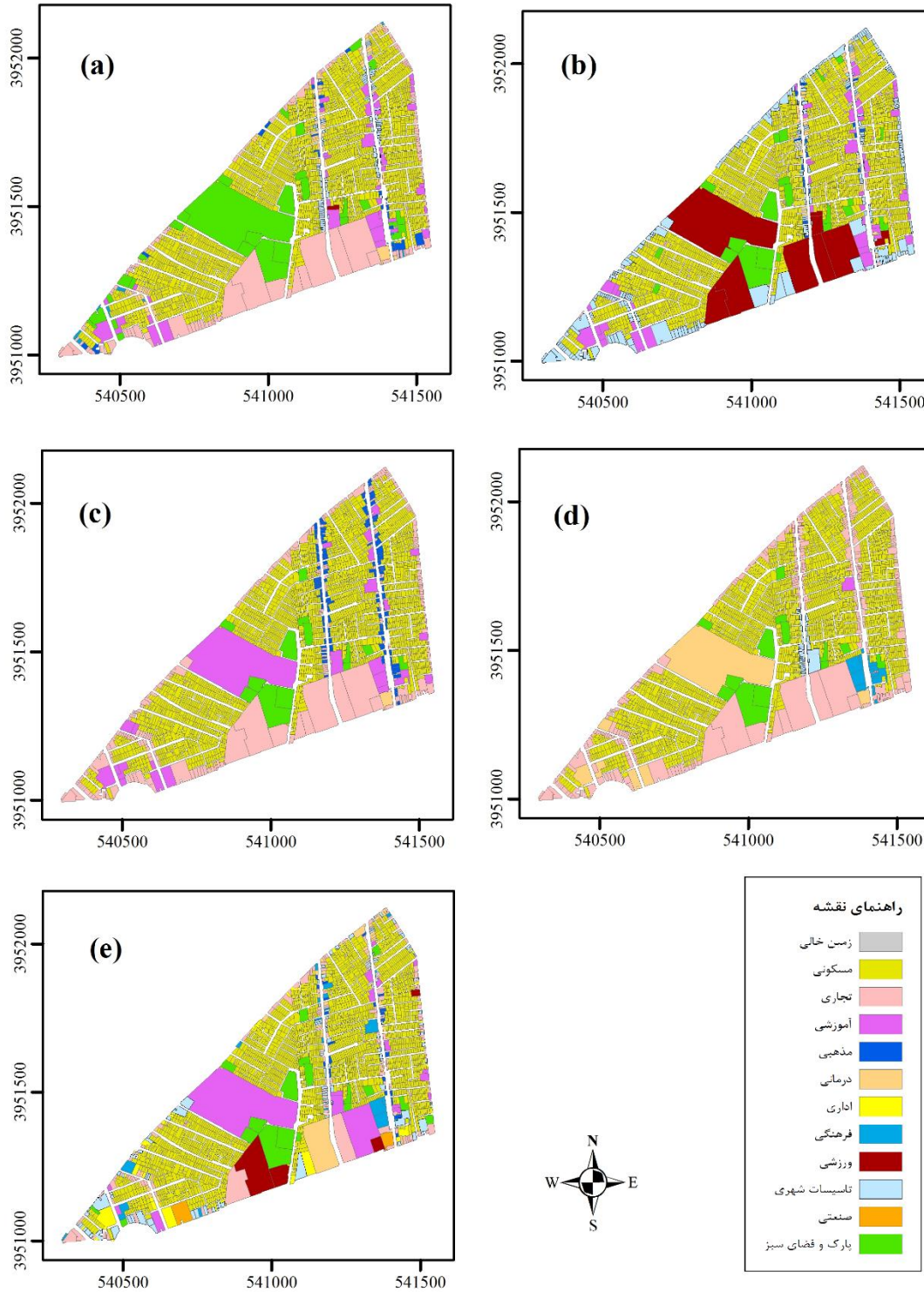
شکل ۹: بهترین چیدمان کاربری‌های با توجه به اهداف مختلف، (a). چیدمان با بیشترین سازگاری، (b). چیدمان با بیشترین وابستگی، (c). چیدمان با بیشترین تناسب، (d). چیدمان با بیشترین همسانی کاربری‌های مجاور، (e). چیدمان با بیشترین تأمین سرانه
