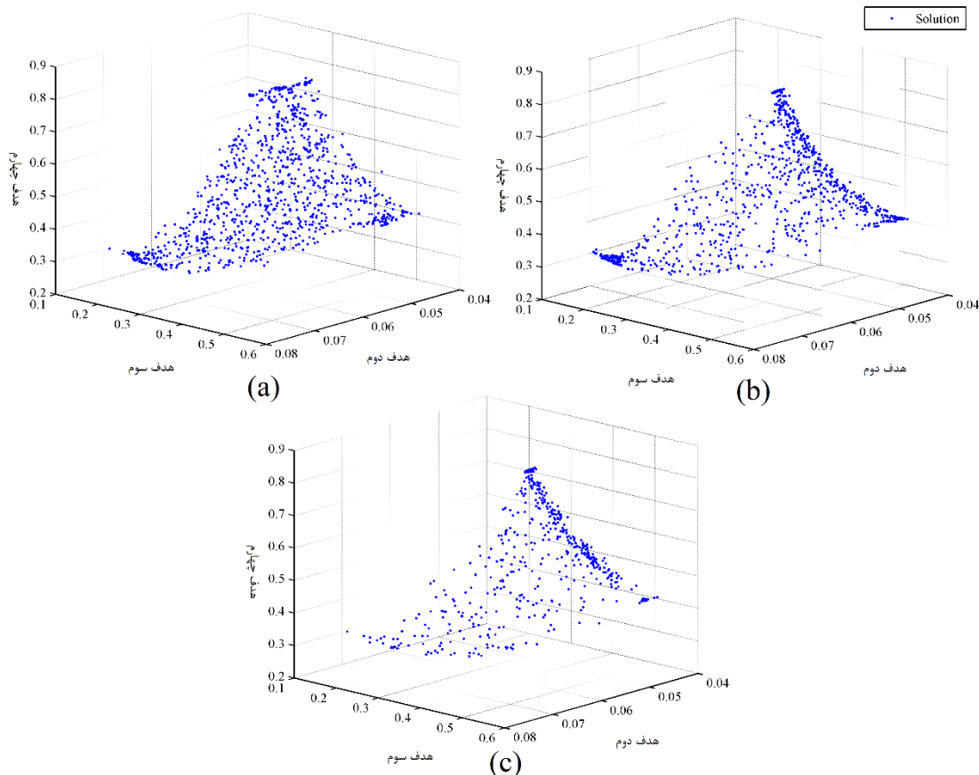
شکل ۱۲: جواب‌های نامغلوب در فضای اهداف (a) جواب‌های حاصل از الگوریتم پیشنهادی. (b) جواب‌های حاصل از الگوریتم NSGAI. (c) جواب‌های حاصل از الگوریتم NSGAIII
